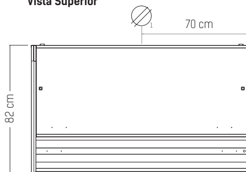
Vista Superior
