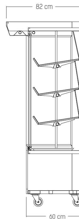
Vista Lateral
